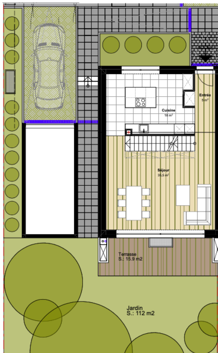
REZ-DE-JARDIN
